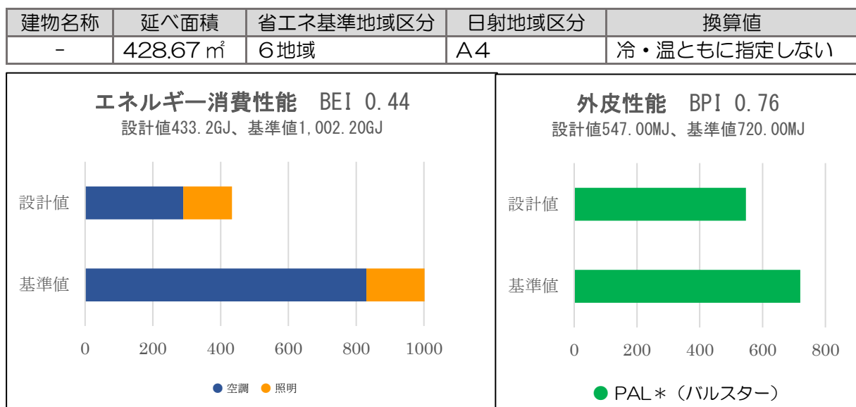
2-40 某物販店事例 出典：ダイキンHVACソリューション九州㈱を元に作成
