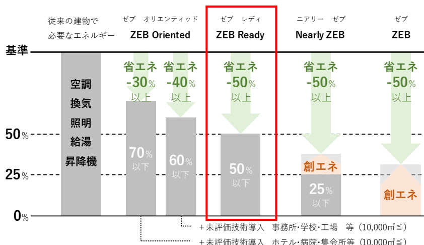
2-38 ZEB シリーズ 出典：ダイキンHVACソリューション九州(株)
