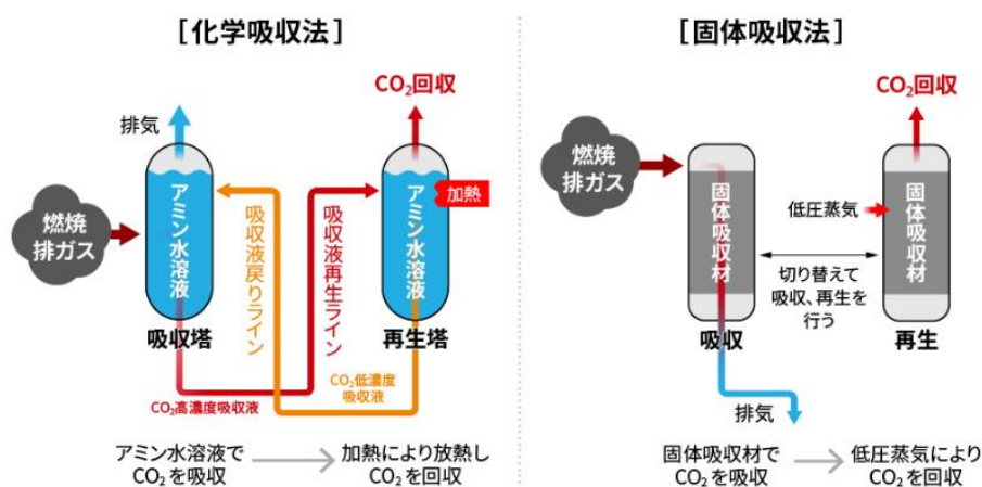
2-70 アミン吸収法 出典：NTT
