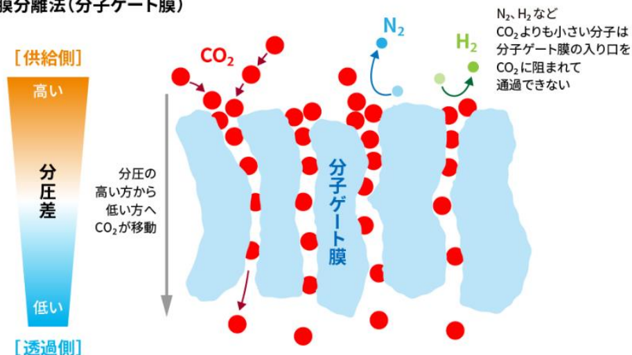
2-72 膜分離法 出典：NTT
