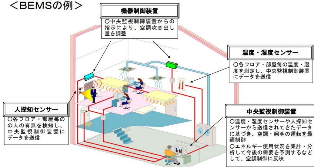
2-41 BEMS の例 出典：環境省
