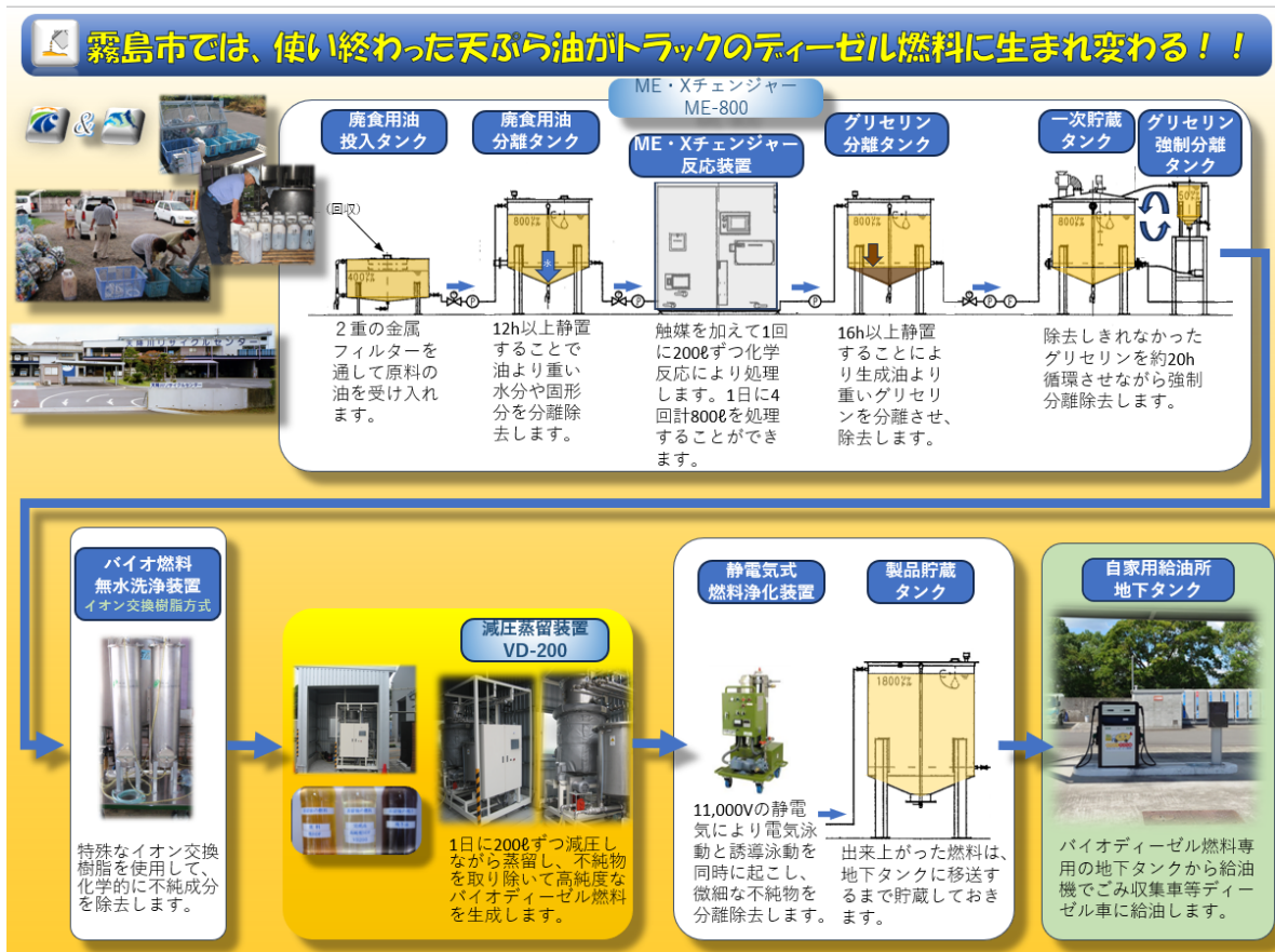
2-61 家庭から出る天ぷら油の回収からトラックのディーゼル燃料に変わるまで 出典：(株)国分集人衛生公社
