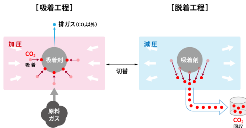
2-71 物理吸着法 出典：NTT
