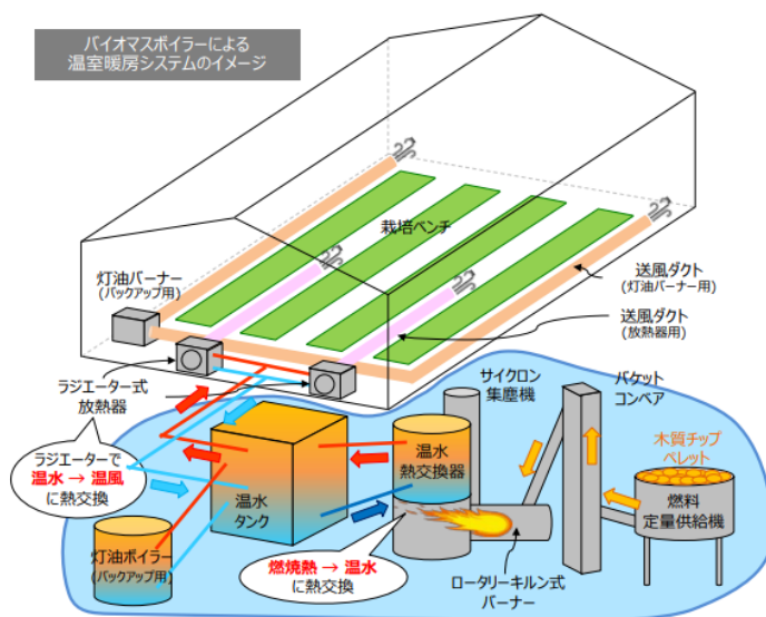
2-21 バイオマスボイラーによる温室暖房システムのイメージ 出典：農研機構
