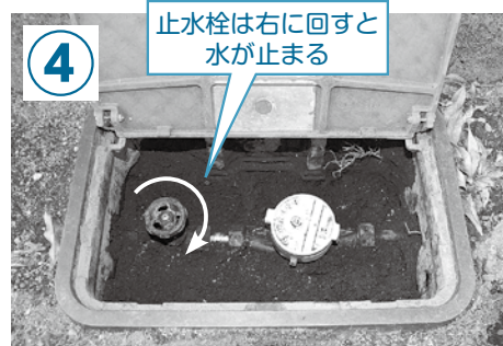
水道メーター器ボックス内の止水栓
