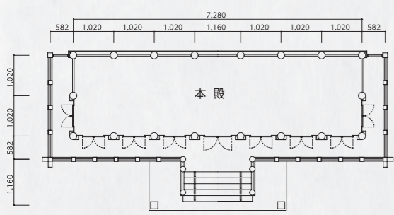
日枝神社本殿の平面図
