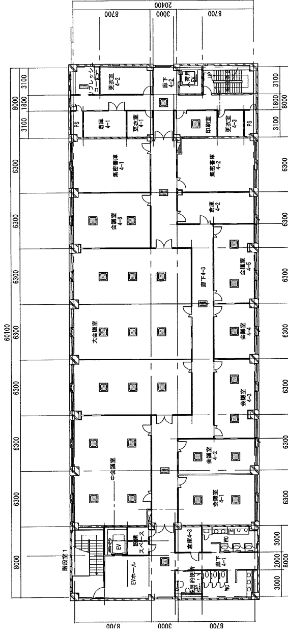
4階平面図
