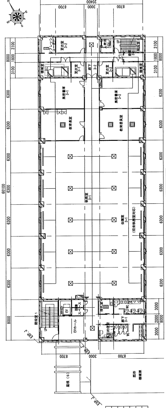
3階平面図
